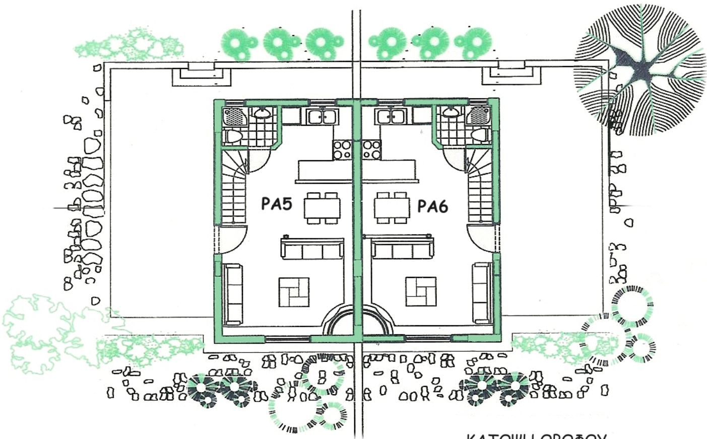
ΚΑΤΟΨΗ ΟΡΟΦΟΥ ΚΑΤΟΙΚΙΩΝ PA5 & PA6
